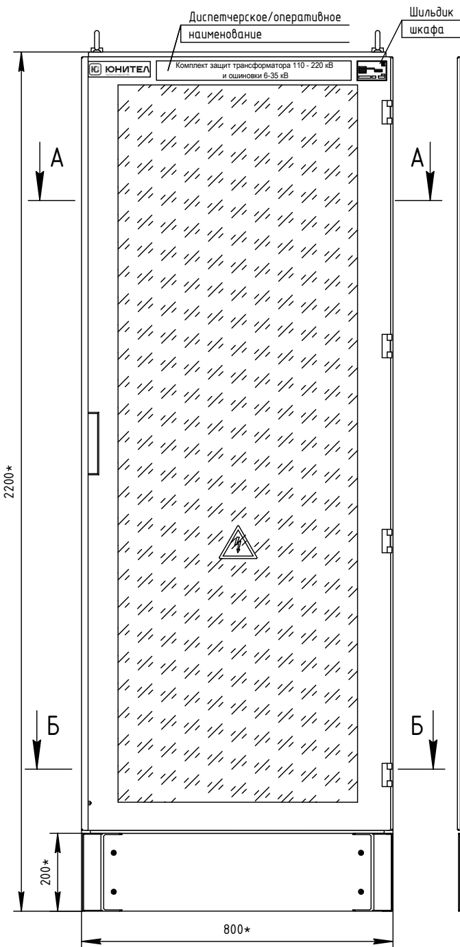
Вид спереди
